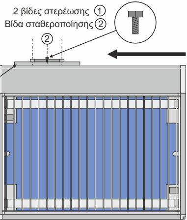
Σχήμα 3. Εμπρόσθια όψη
